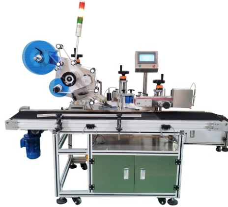
| 全自动平面侧面一体贴标机 |
